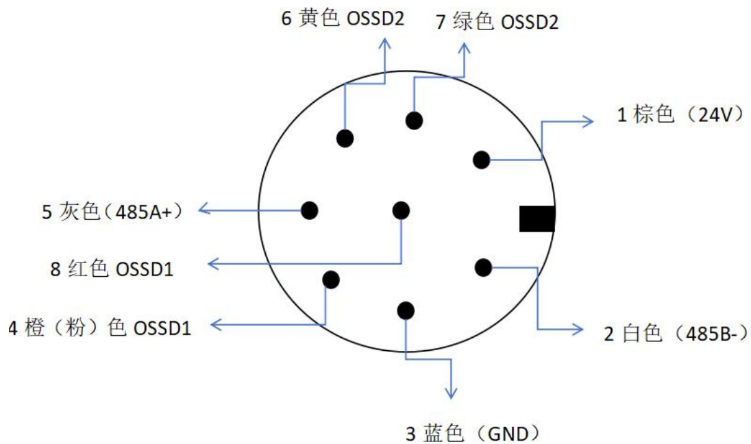
图 10 雷达接口引脚定义图
