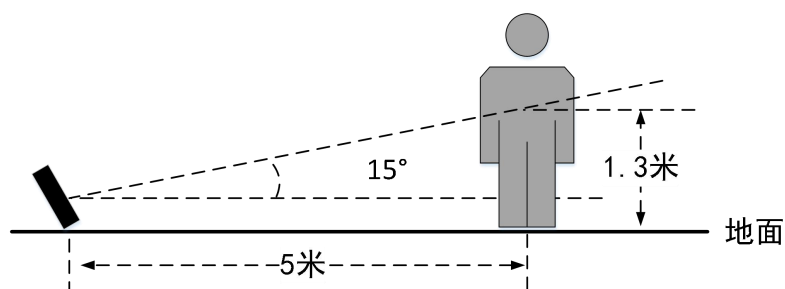
图 4 安装在地面：俯仰角 15^{\circ}
