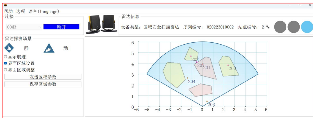
图 24 软件界面
