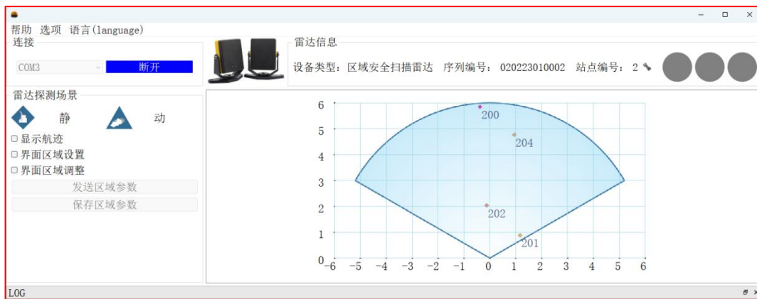
图 23 软件界面
