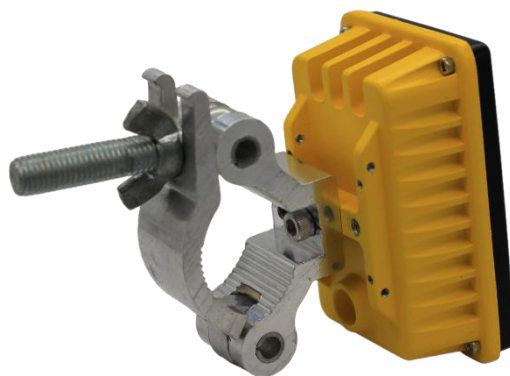
图 2 雷达安装侧视图
